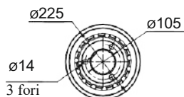
sez. A-A
